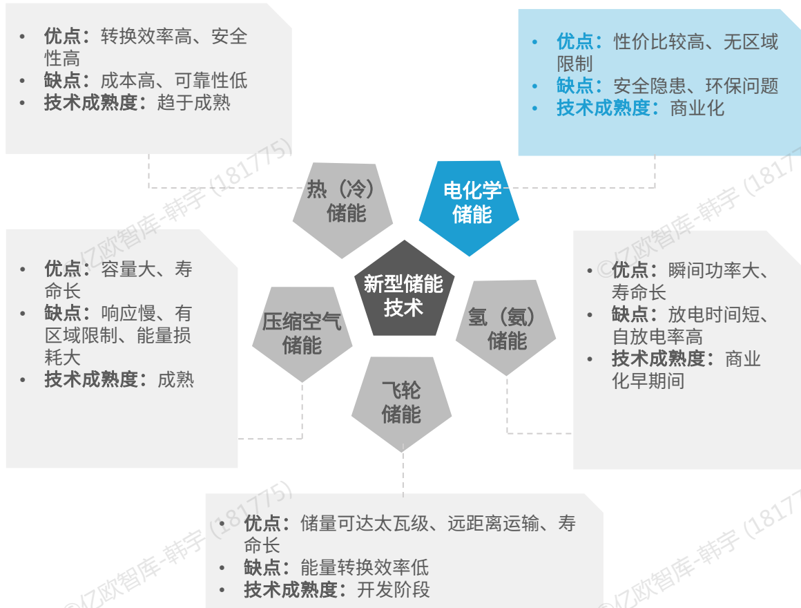
亿欧智库：主要新型储能技术对比
