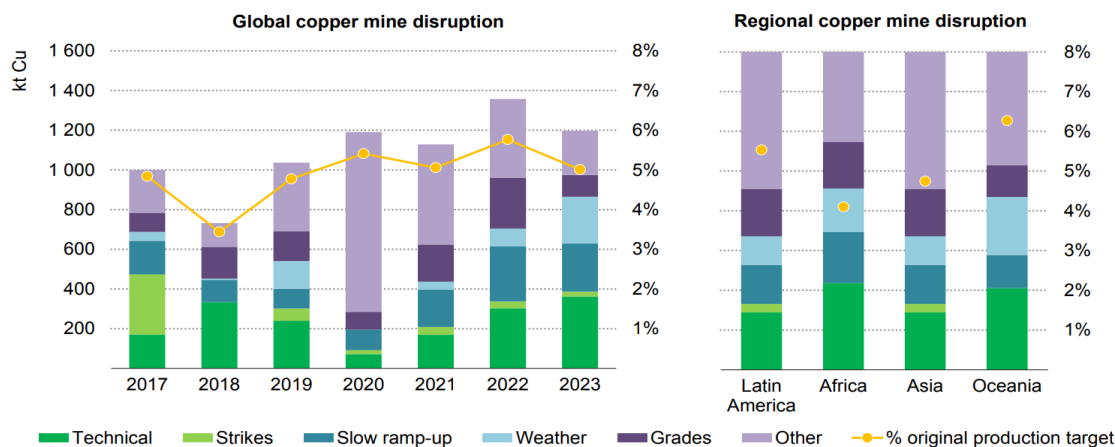
图36：全球铜矿扰动频发
