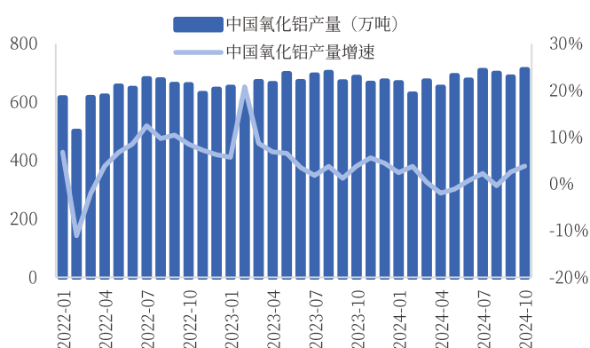
图77: 国内氧化铝产量及产量增速
