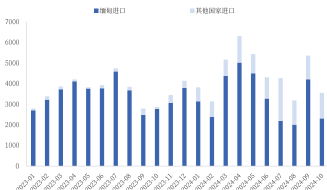
图93：2023-2024 年 10 月我国进口未列明稀土氧化物情况（吨）
