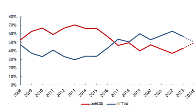
图42: 废铜流向冶炼端比例抬升
