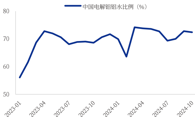
图71: 国内电解铝行业铝水直接合金化比例
